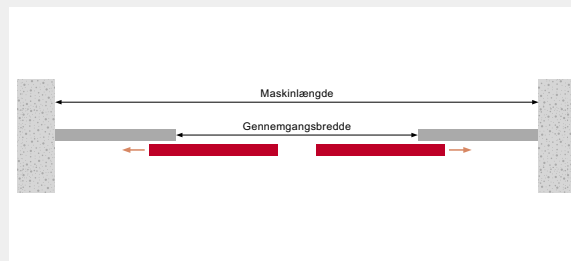
Plan snit (dobbeltfløjet, med faste sidepartier)
